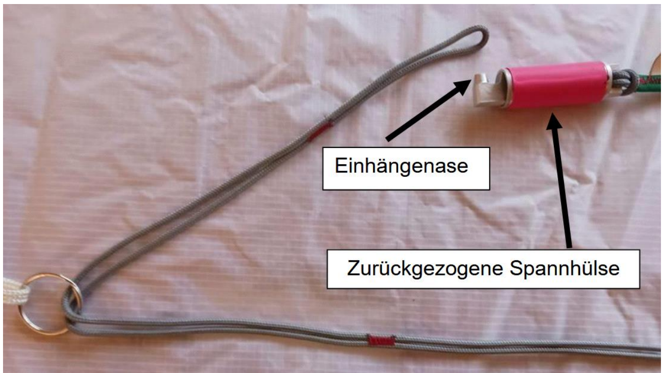
Abbildung 5.1: Spannhülse zurückgezogen
