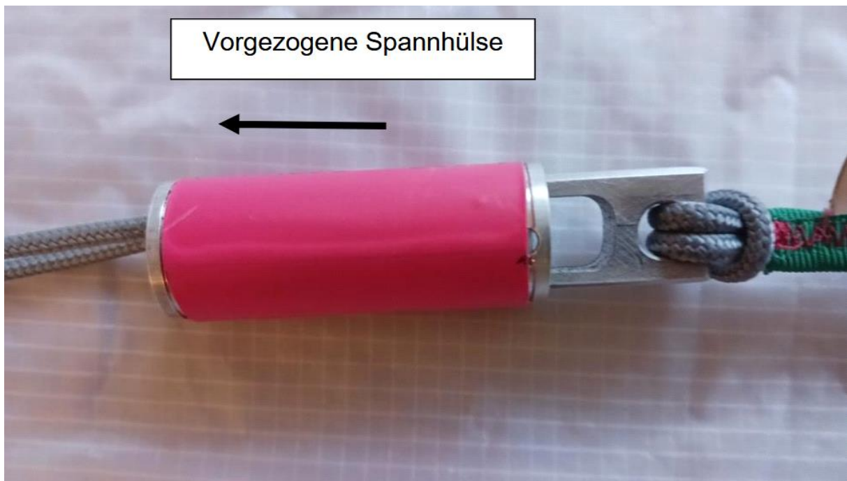
Abbildung 5.3: Schleppklinke im startbereiten Zustand
