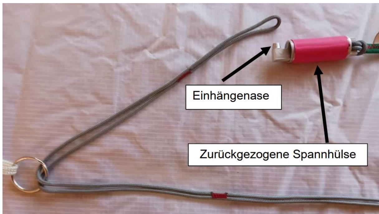
Abbildung 5.1: Spannhülse zurückgezogen
